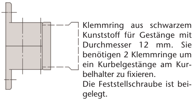
Klemmring Best. Nr.- 5186.10-0001
