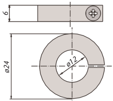
Klemmring Best. Nr.- 5186.10-0001
