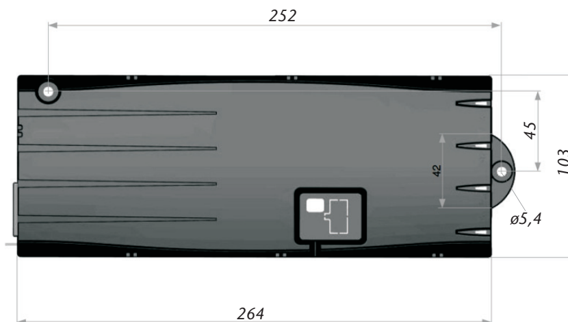
Steuerung Compact-3
